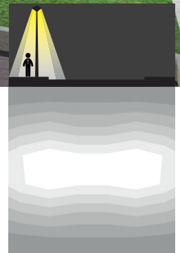
A2 - symmetrisch smalstralend
